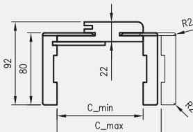
Przekrój ORB 075
