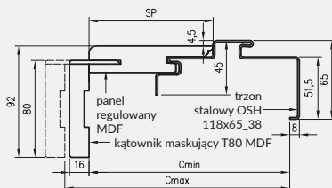
profil ościeżnicy
